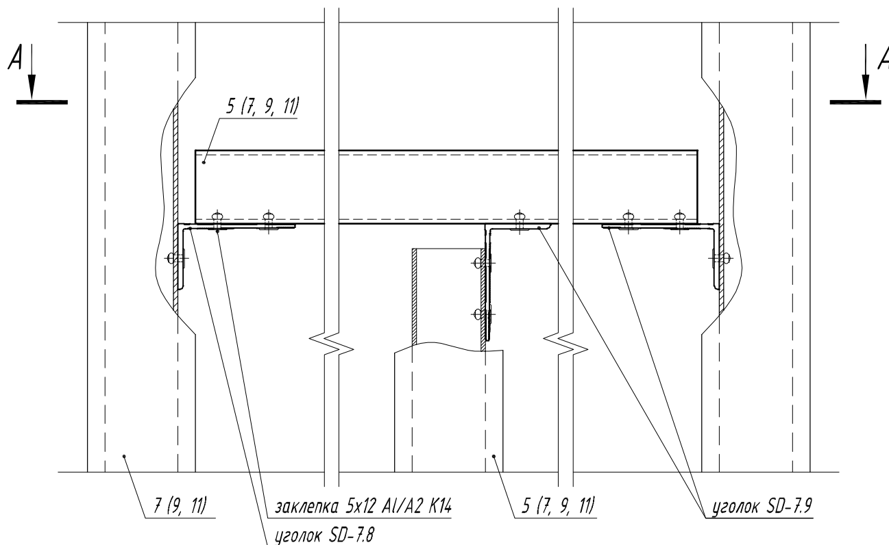
Вид В
